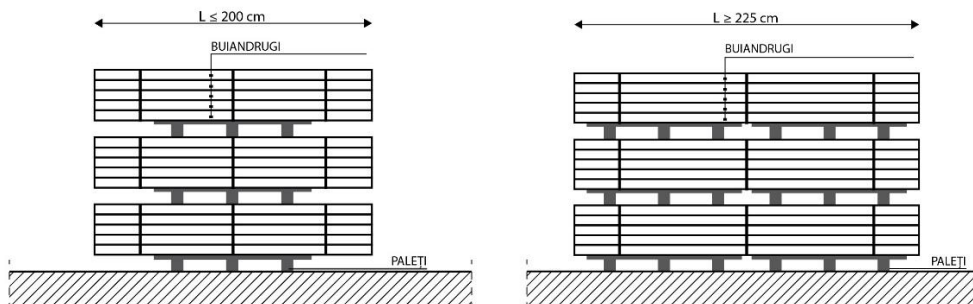
Modul de depozitare pe paleti a buiandrugilor Cemacon 115X69
